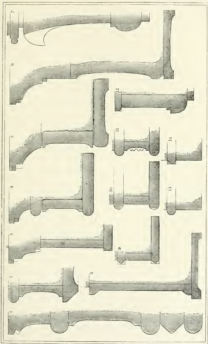
PLATE VIII.—BYZANTINE ARCHIVOLTS
